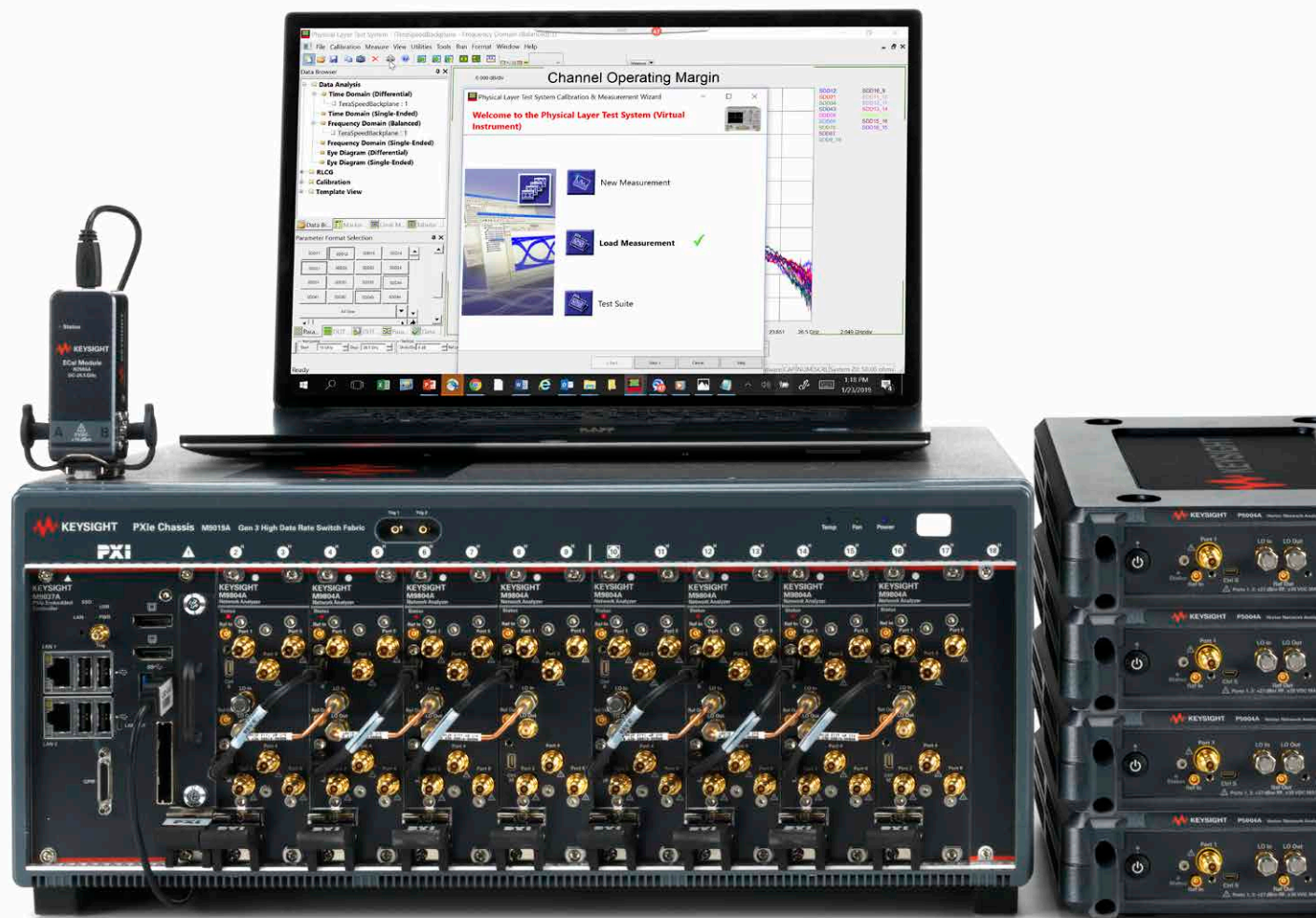
装有 M9804A PXI 矢量网络分析仪的 M9019A PXI 机箱
